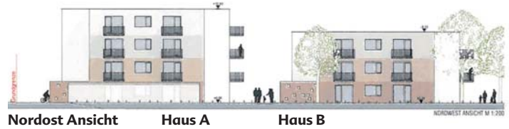
Nordost Ansicht Haus A Haus B NORDWEST ANSICHT M 1:200
